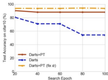
CIFAR10
