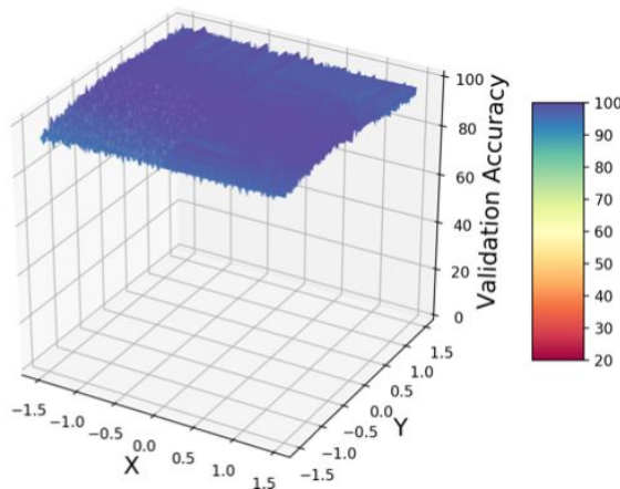
(b) SDARTS-RS
