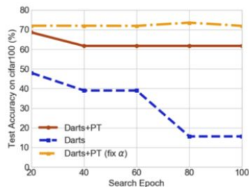
CIFAR100
